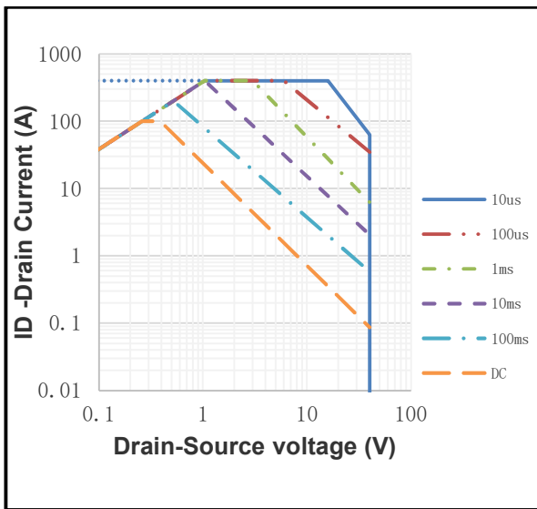
Fig.13 SOA
